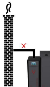
Lang afstand mellem kedel og skorsten = kuldebro og højt modtryk.
