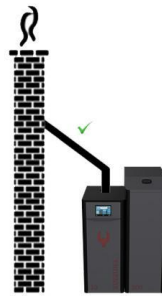
Længere afstand mellem kedel og skorsten kan med fordel laves med 45° knæk.
