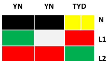
Tilslutning motorprint MOTOR (12 PIN)
